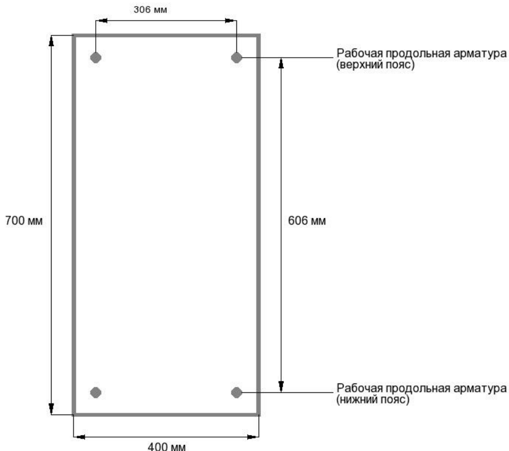
Расположение продольной арматуры по сечению ленты
